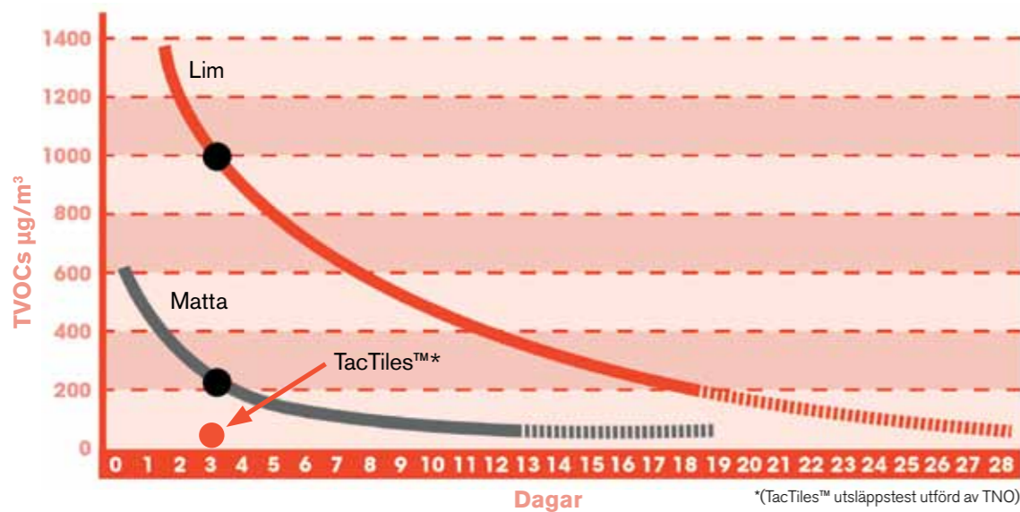
Typisk utsläppskurva för lim och installation
